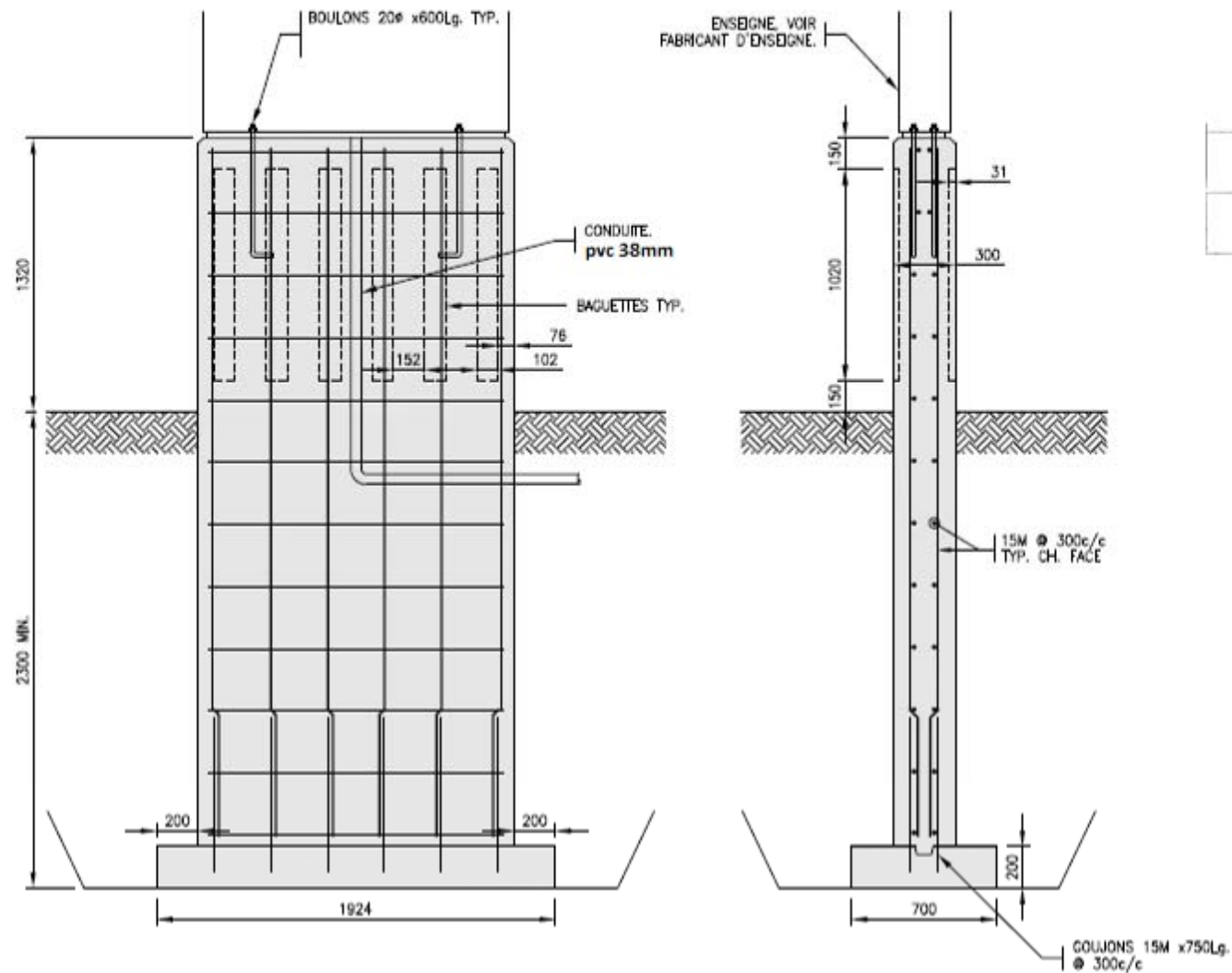
DÉTAIL TYPE - BASE POUR ENSEIGNE
